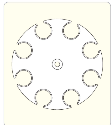
分液ロート架板形状
